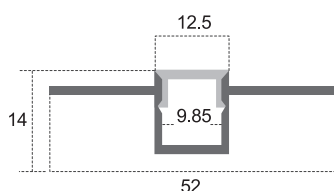
CL-Alu-7030 UD
